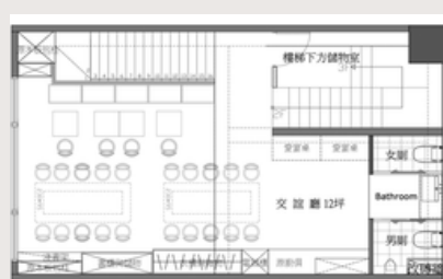
新教堂二樓副堂、三樓辦公室及教室設計初稿
